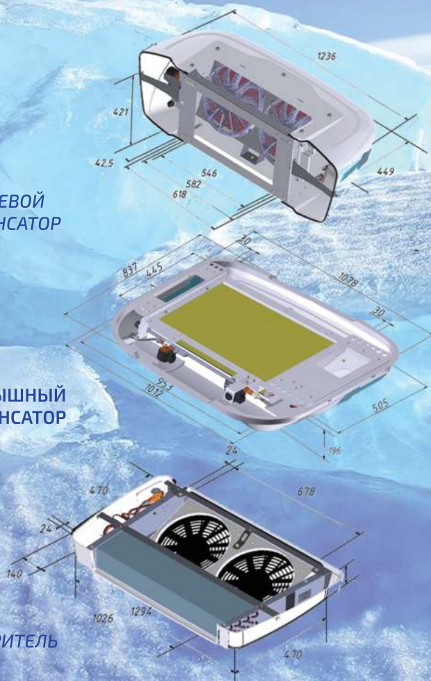
ИСПАРИТЕЛЬ
